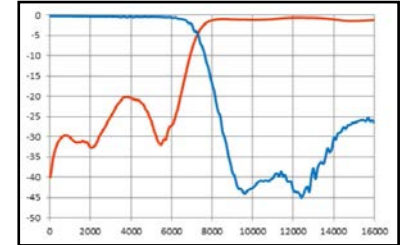
0805 size, 6 GHz LPF 8W
