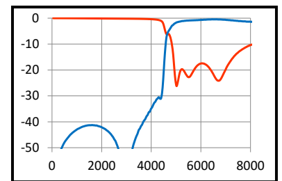
0805 size, 5.15 GHz HPF 5W
