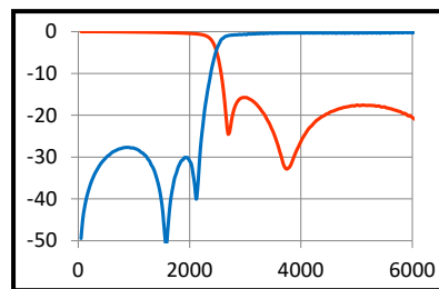
0805 size, 2.7 GHz HPF 5W
